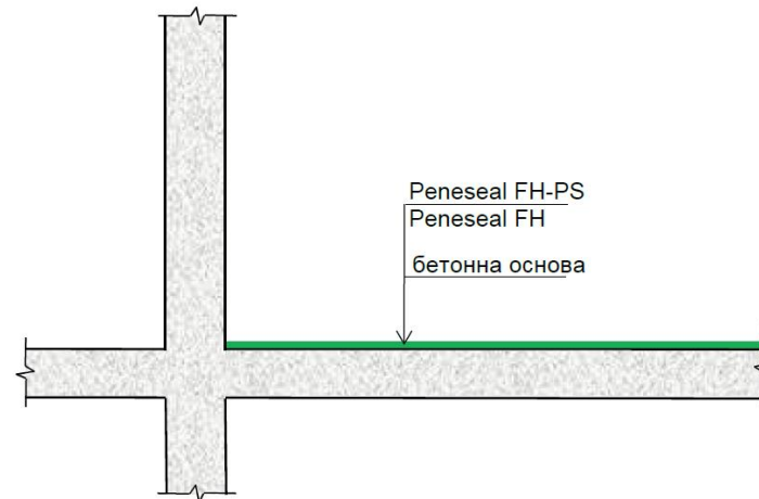
Рисунок I-13-1. Стандартна схема улаштування зносостійких підлогових покриттів для приміщень м'ясо-переробної промисловості
