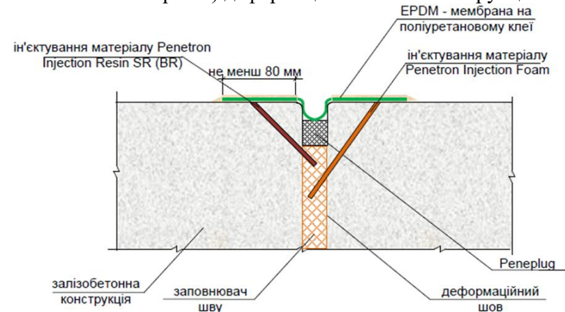
Рисунок I-12-2. Схема улаштування герметизації протікаючих (на момент виконання робіт) деформаційних швів конструкцій, що передбачають рухомі з'єднання елементів
