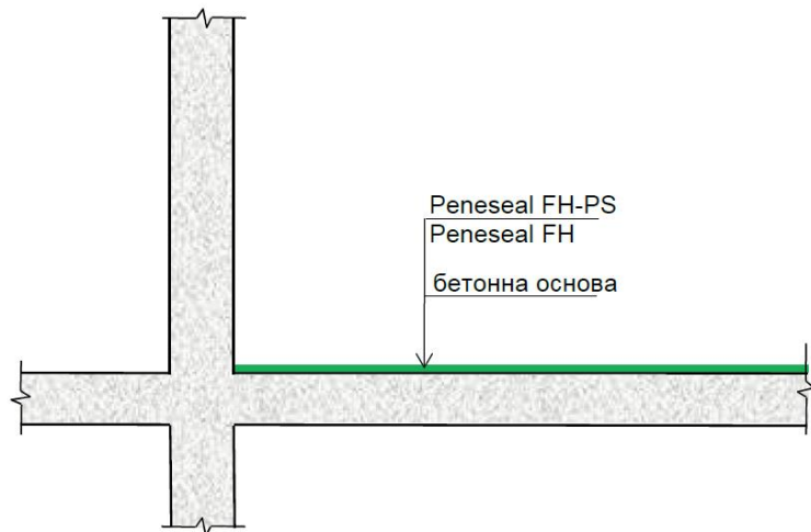
Рисунок П-15-1. Схема відновлення зносостійких підлогових покриттів для приміщень агропромислового комплексу
