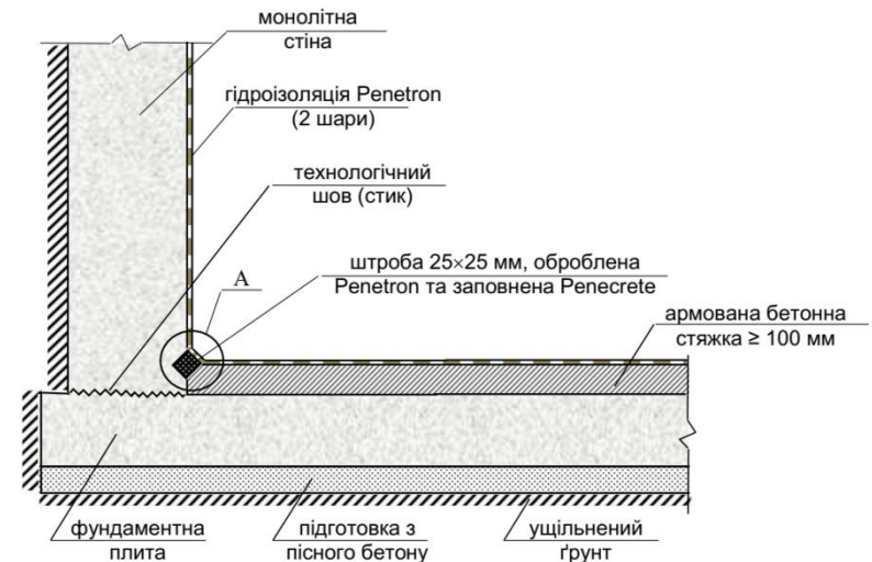
Рисунок 1 Приклад стандартної схеми конструкції із застосуванням Penetron.
