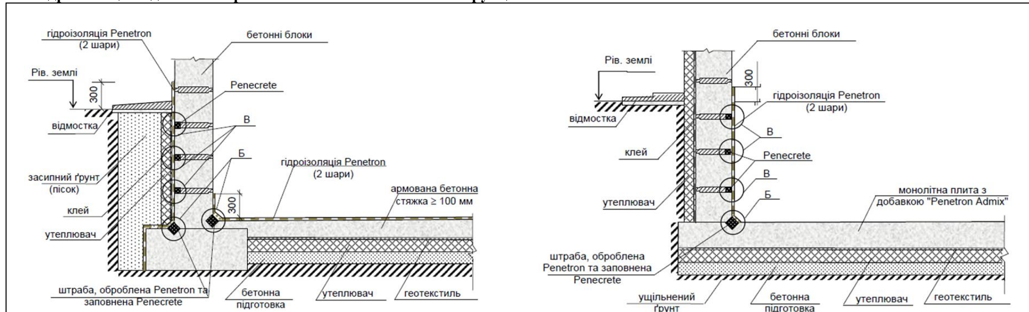
Рисунки I-8-1 і I-8-2. Схеми улаштування гідроізоляції підземних внутрішніх і зовнішніх поверхонь збірних елементів конструкцій та монолітних бетонних основ
