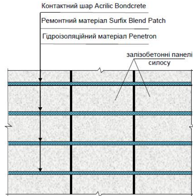
Рисунок П-7-2. Схема відновлення стиків між збірними елементами огорожувальних залізобетонних конструкцій
