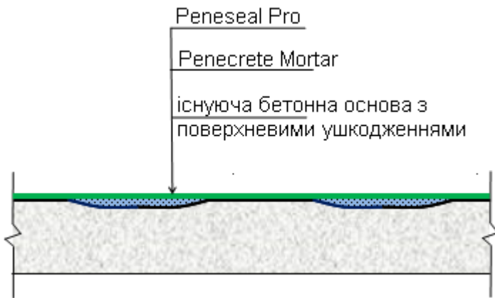
Рисунок П-19-1. Стандартна схема зміцнення існуючих бетонних основ, що експлуатуються під впливом навколишнього середовища
