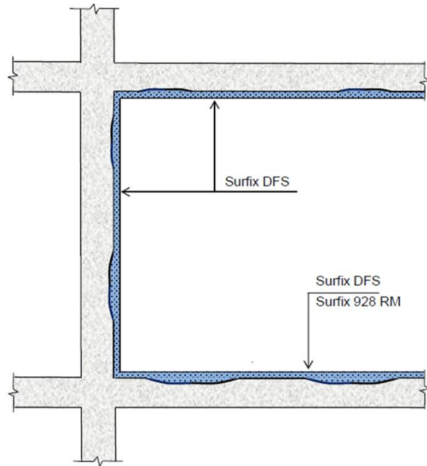
Рисунок П-13-1. Схема відновлення бетонних поверхонь холодильних приміщень із застосуванням гідроізолюючих ремонтних матеріалів Surfix™
