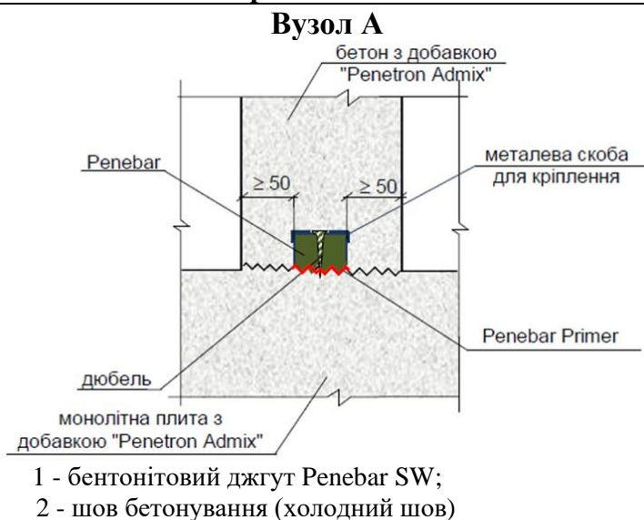
Рисунок I-4-1. Схема розташування швів бетонування та монтажу бентонітового джгута Penebar SW
