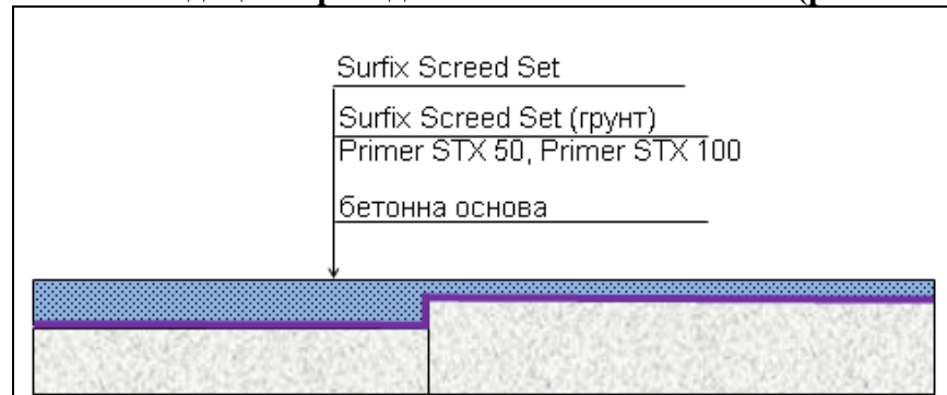
Рисунок П-20-1. Стандартна схема ліквідація перепадів висотного положення (рівнів чистої підлоги) бетонних підлог суміжних приміщень
