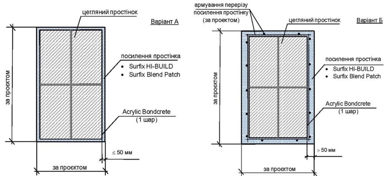
Рисунки П-8-2 і П-8-3. Схеми посилення простінків з цегляної кладки
