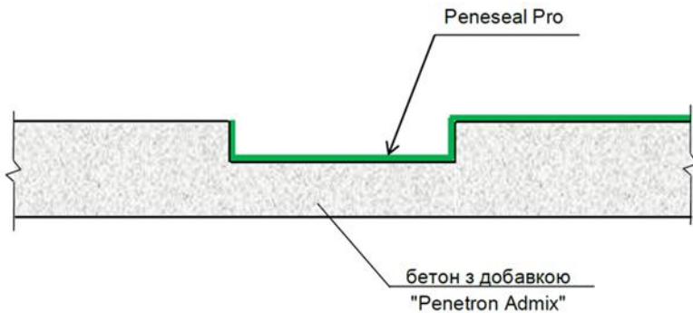
Рисунок I-19-1. Стандартна схема антикорозійного захисту конструкції лоткової системи для видалення гною з будівлі тваринницької ферми
