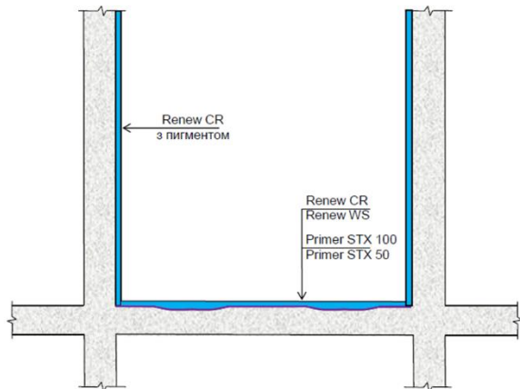
Рисунок П-14-1. Схема відновлення естетичного вигляду та структурної міцності бетонних поверхонь стін та підлог складських і виробничих приміщень
