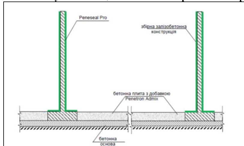
Рисунок I-17-1. Стандартна схема антикорозійного захисту збірних і монолітних конструкцій секційних силосних траншей на території тваринницьких комплексів
