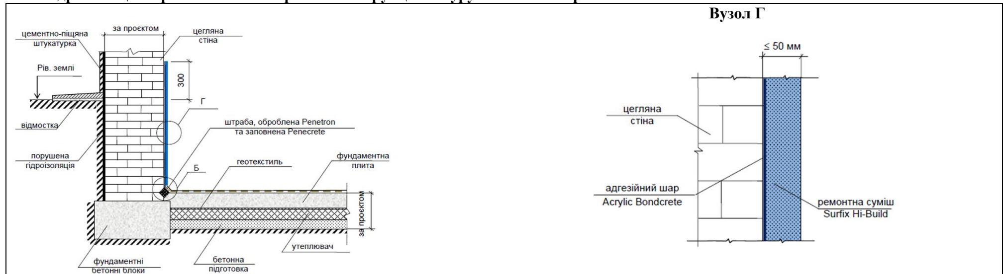
Рисунок П-3-1. Схема улаштування внутрішньої гідроізоляції вертикальних поверхонь конструкцій із мурувальних матеріалів (без капілярного підсмоктування)
