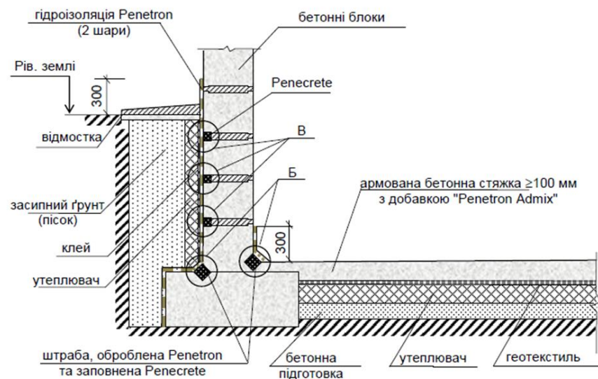
Рисунки П-2-4 і П-2-5. Схеми улаштування зовнішньої і внутрішньої гідроізоляції збірних конструкцій стін та фундаментних плит
