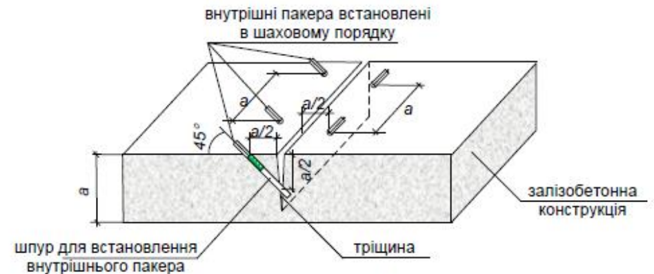
Рисунок II-9-3. Схема розташування ін'єкційних пакерів для герметизації порожнин та водоненасичених статичних тріщин
