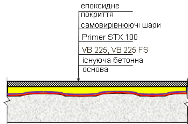
Рисунок П-16-1. Стандартна схема відновлення бетонних підлог, що експлуатуються в умовах накопичення відходів життєдіяльності тварин
