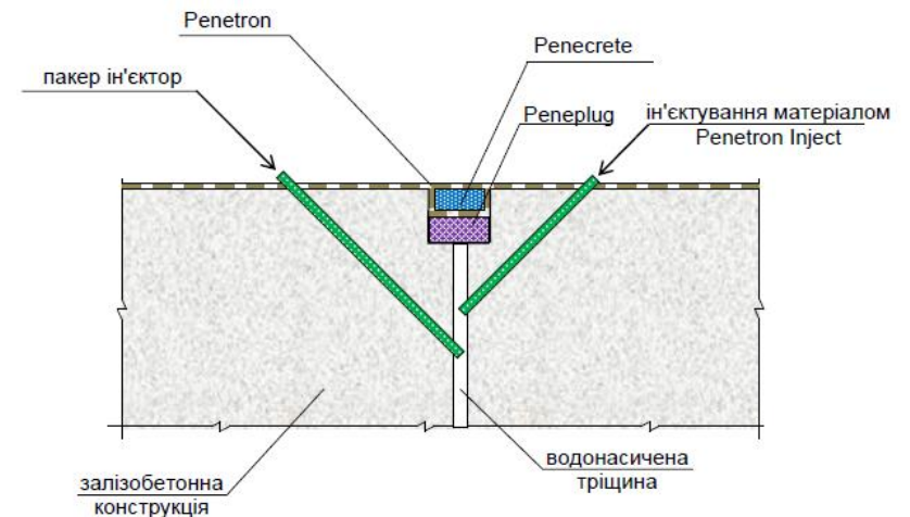
Рисунок П-10-2. Схема герметизації водонасиченої статичної тріщини шириною розкриття понад 0,5 мм під дією гідростатичного тиску
