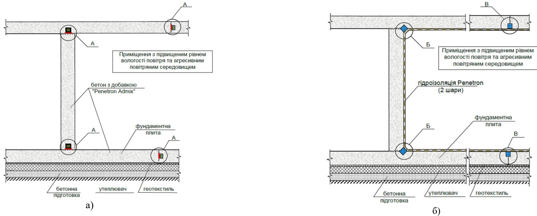
Рисунки I-10-1 і I-10-2. Схеми улаштування гідроізоляції внутрішніх приміщень із застосуванням щільного бетону з добавкою в бетон Penetron Admix (а) та гідроізоляційного матеріалу проникаючої дії Penetron (б)
