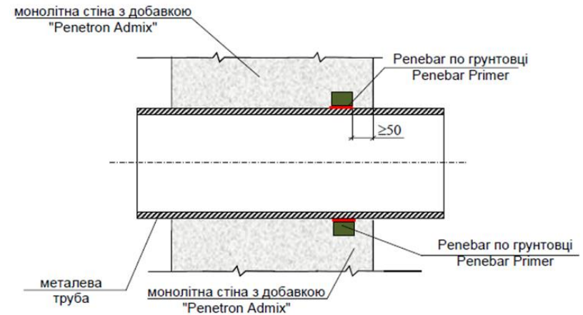
Рисунок I-6-2. Схема гідроізоляції місця вводу комунікаційної труби з гільзою типу «бетон – гільза»
