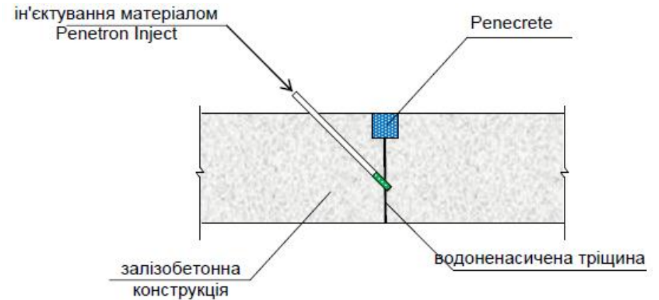
Рисунок II-9-2. Схема ін'єктування порожнин та водоненасичених статичних тріщин
