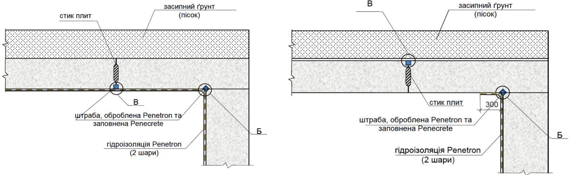
Рисунки I-9-1 і I-9-2. Схеми улаштування гідроізоляції підземних горизонтальних поверхонь збірних елементів конструкцій перекриття
