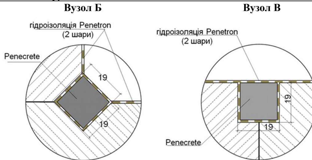
Рисунки I-5-3 і I-5-4. Схеми улаштування гідроізоляції стиків і примикань збірних елементів конструкцій
