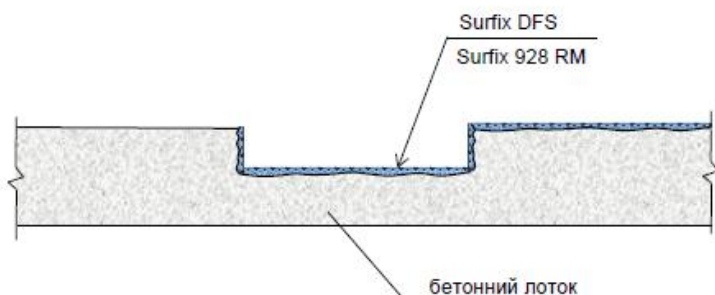
Рисунок П-17-1. Схема відновлення бетонних поверхонь лоткової системи для видалення гною з будівлі тваринницької ферми із застосуванням гідроізолюючих ремонтних матеріалів Surfix™
