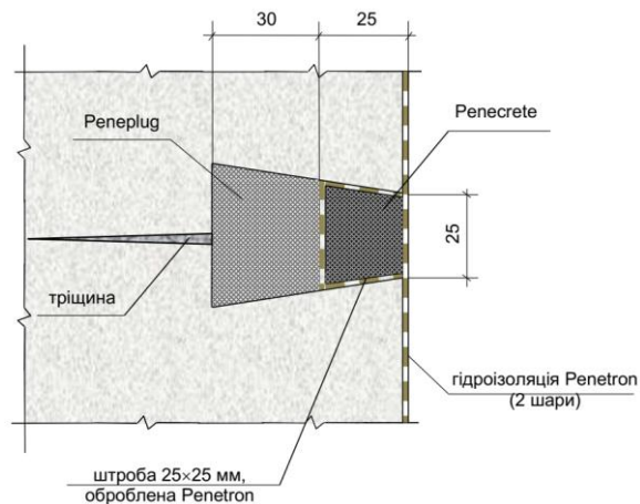
Рисунок 1 Приклад стандартної схеми конструкції із застосуванням Реперplug
