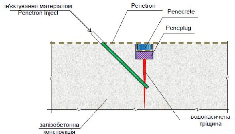
Рисунок П-9-4. Схема ін'єктування водонасиченої статичної тріщини шириною розкриття понад 0,5 мм
