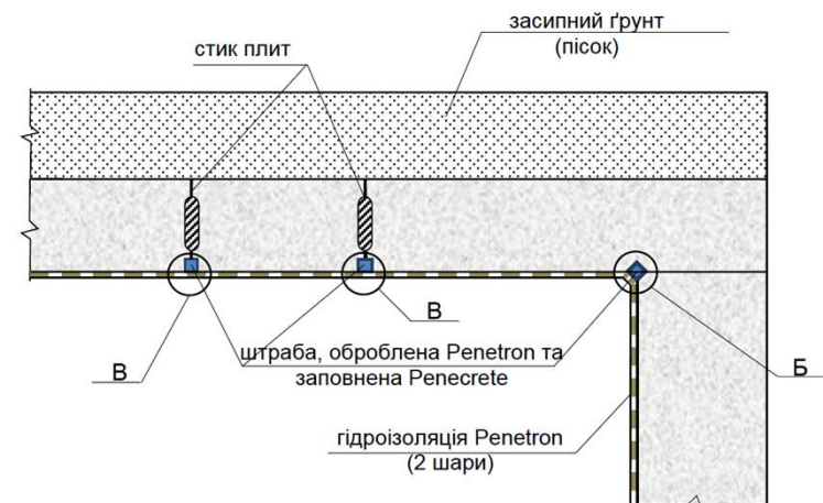
Рисунки II-2-2 і II-2-3. Схеми улаштування внутрішньої гідроізоляції збірних конструкцій стін і перекриття та фундаментних плит
