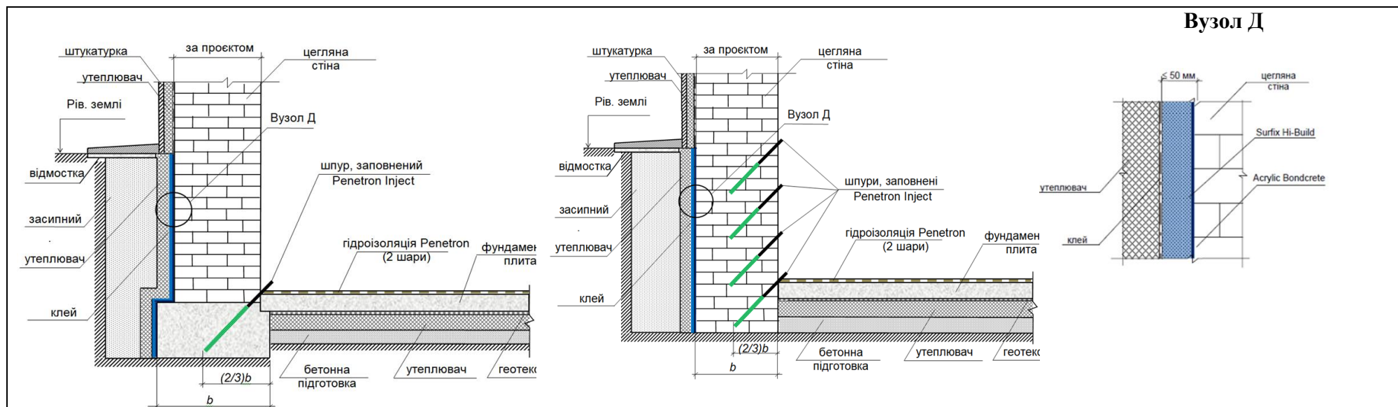
Рисунки П-3-2 і П-3-3. Схеми улаштування зовнішньої та внутрішньої гідроізоляції вертикальних поверхонь конструкцій із мурувальних матеріалів (з відсіканням капілярного підсмоктування)
