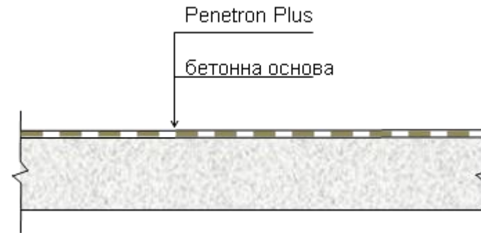
Рисунок I-14-1. Стандартна схема конструкції зносостійкої підлоги з підвищеним рівнем стійкості до ударів та стирання
