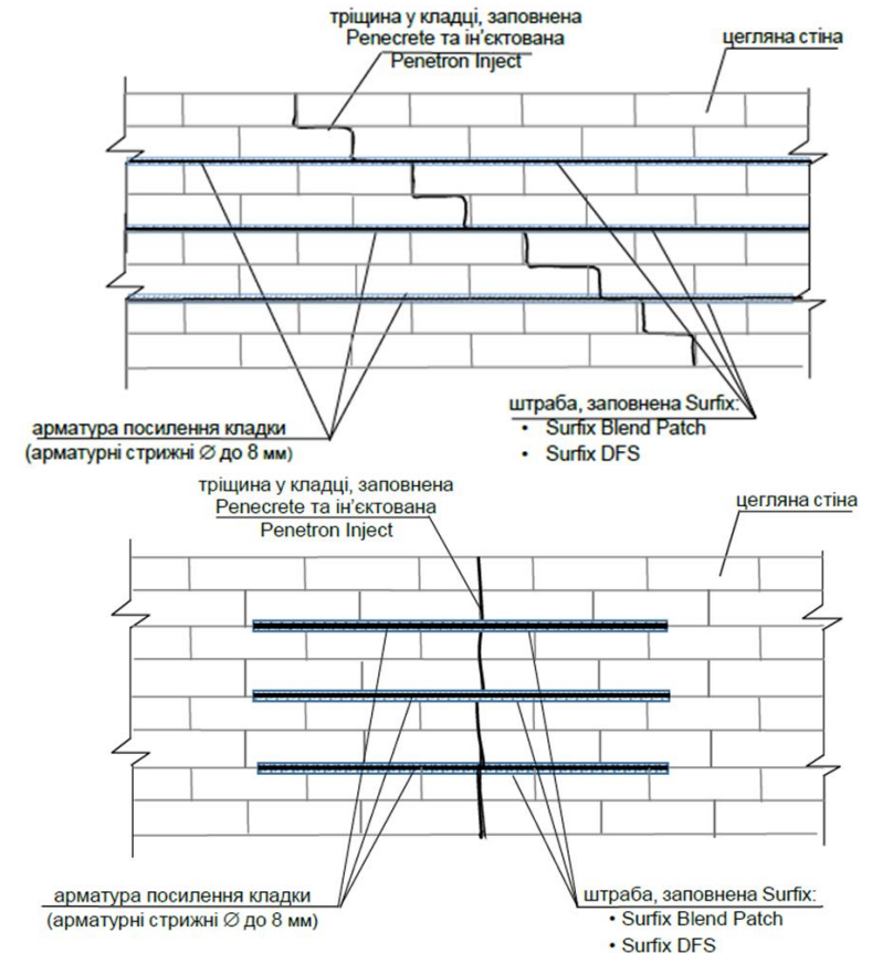
Рисунок П-8-5. Схеми посилення кладки цегляної стіни з похилими та вертикальними тріщинами
