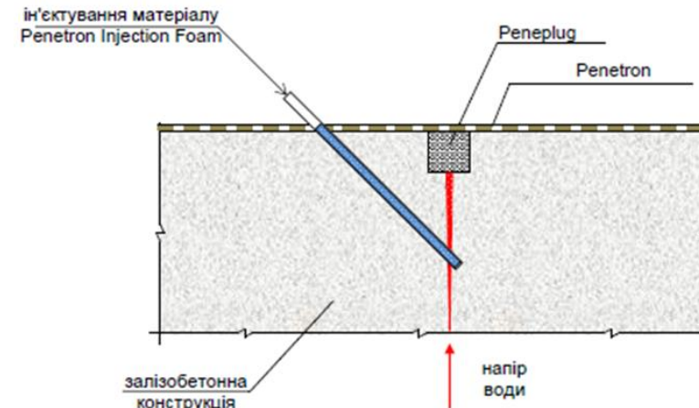
Рисунок П-11-1. Схема улаштування герметизації обмежено рухомих протікаючих тріщин
