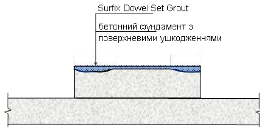
Рисунок П-21. Стандартна схема відновлення бетонного фундаменту з поверхневими ушкодженнями під стаціонарне технологічне устаткування
