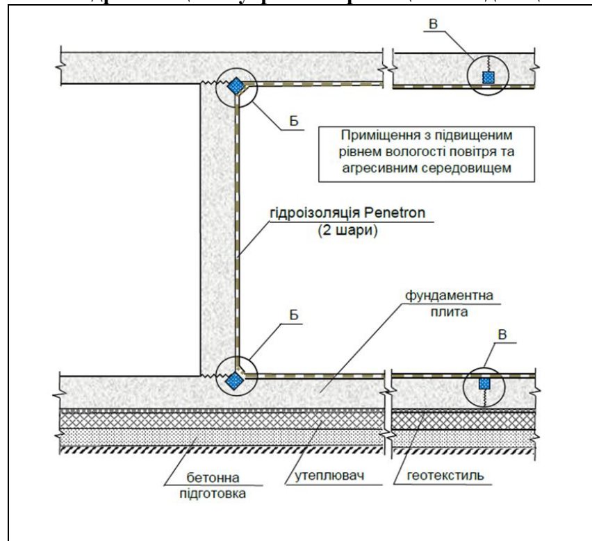
Рисунок П-12-1. Схема влаштування гідроізоляції внутрішніх приміщень із застосуванням гідроізоляційного матеріалу проникаючої дії Penetron
