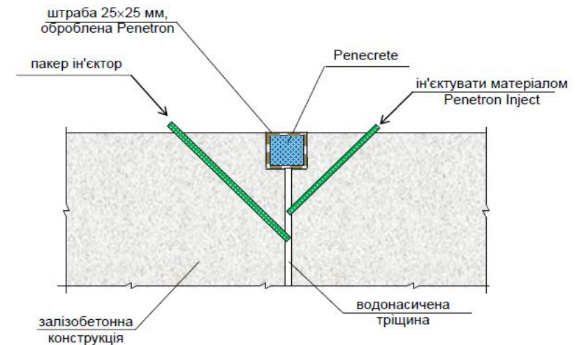
Рисунок П-10-1. Схема герметизації водонасиченої статичної тріщини шириною розкриття понад 0,5 мм без гідростатичного тиску
