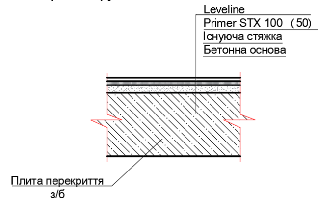
Рисунок 1 Приклад стандартної схеми конструкції із застосуванням матеріалів групи Leveline
