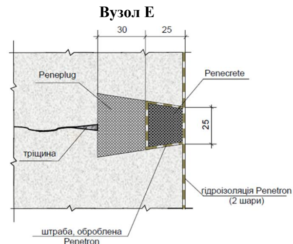
Рисунок П-9-5. Вузол Е при ін'єктуванні водонасиченої статичної тріщини шириною розкриття понад 0,5 мм
