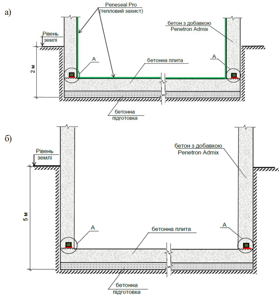
Рисунки I-16-1 і I-16-2. Стандартна схема антикорозійного захисту конструкції секційних карантинних ємностей (а) і секційних гноєсховищ (б) на території тваринницьких комплексів
