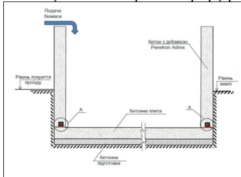
Рисунок I-18-1. Стандарта схема антикорозійного захисту бетонних приймальних резервуарів біогазових установок
