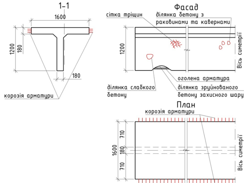
Рисунок III-1-2. Характерні пошкодження балок, що знаходилися в експлуатації
