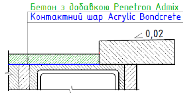
Рисунки П-1-3 і П-1-4. Конструктивні схеми улаштування нової монолітної плити проїзної частини
