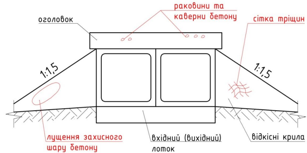
Рисунок IV-4-2. Характерні пошкодження бетонних поверхонь оголовка та відкисних крил труби дорожньої
