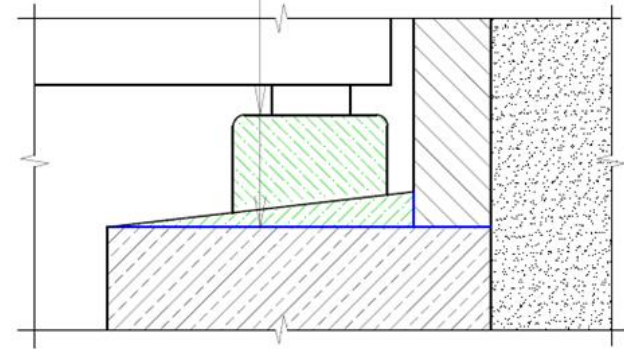
Рисунок I-4-2. Конструктивні схеми улаштування гідроізоляції підферменників та стічних трикутників
