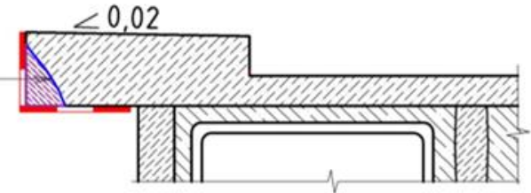
Рисунок П-4-2. Конструктивна схема відновлення бетону захисного шару тротуарних консолей
