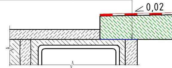
Рисунки II-2-2 і II-2-3. Конструктивні схеми улаштування нових монолітних тротуарів
