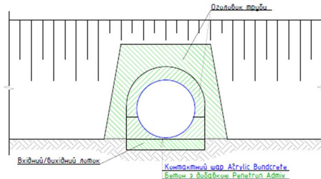
Рисунок IV-2-2. Конструктивна схема влаштування лотків та оголовків труби
