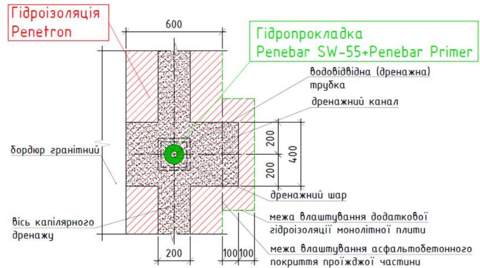
Рисунок I-3-2. Конструктивна схема влаштування гідроізоляції капілярного дренажу
