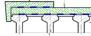
Рисунок I-1-3. Конструктивна схема монолітної плити і монолітного тротуара
