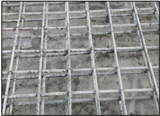
Рисунок I-1-2. Контактний (адгезійний) шар для антикорозійного захисту арматурних сіток та підвищення адгезії до бетону плити прогонових будов і арматури монолітної плити
