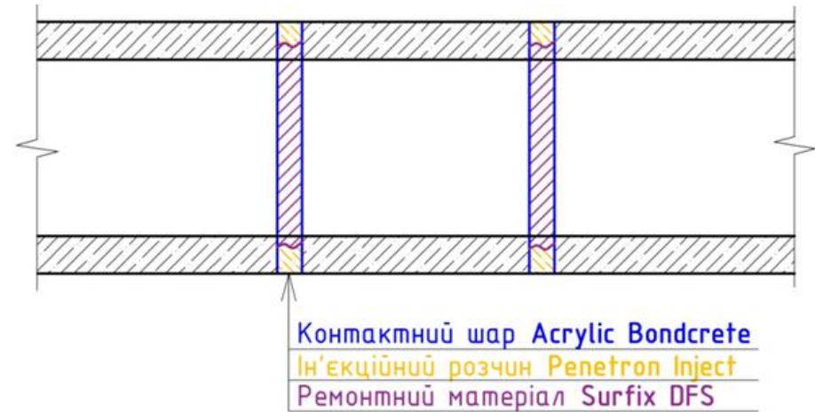
Рисунок IV-3-2. Конструктивна схема відновлення щільності швів між ланками труби
