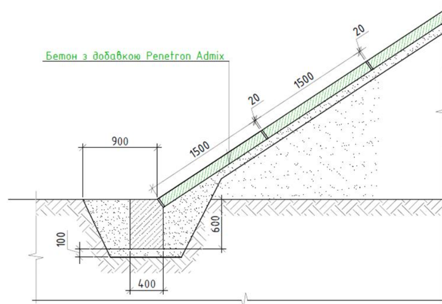
Рисунок I-5-2. Конструктивна схема влаштування гідроізоляції бетонного укріплення конуса насипу
