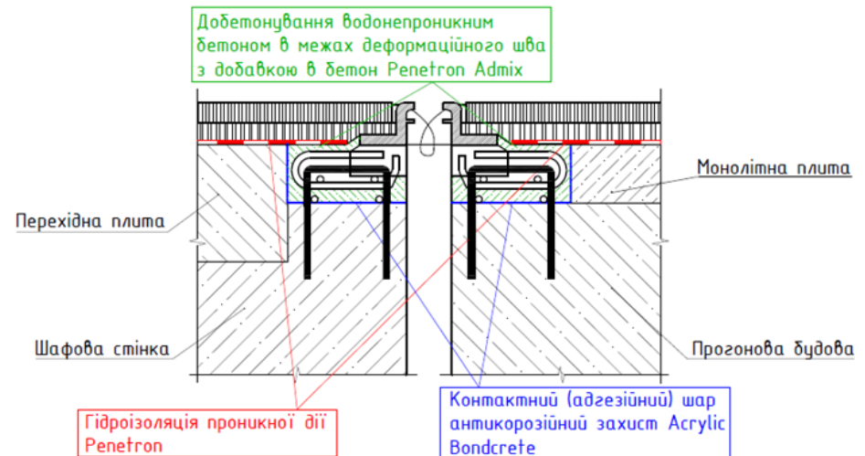
Рисунок П-3-3. Конструктивна схема улаштування гідроізоляції в зоні деформаційного шва
