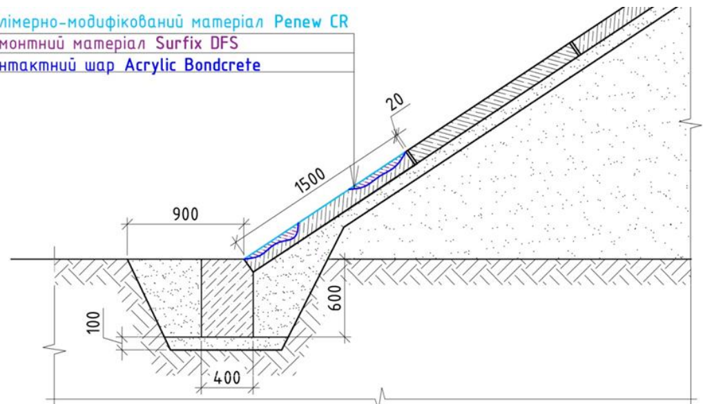
Рисунок П-5-3. Конструктивна схема відновлення бетонного укріплення конуса
