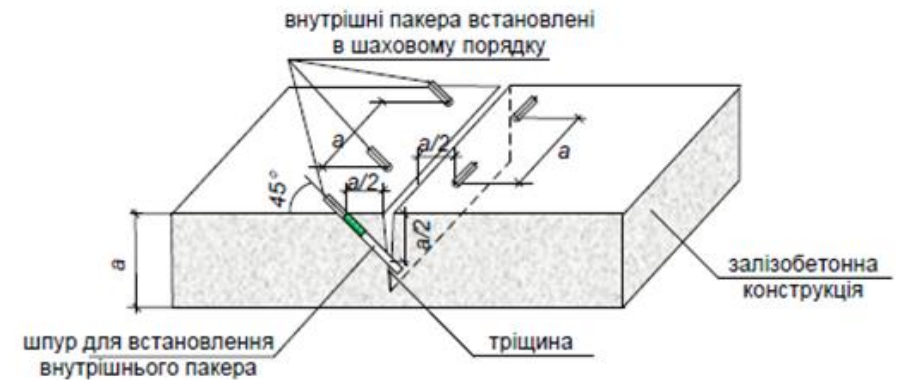
Рисунок П-9-3. Схема розташування ін'єкційних пакерів для герметизації порожнин та водоненасичених статичних тріщин
