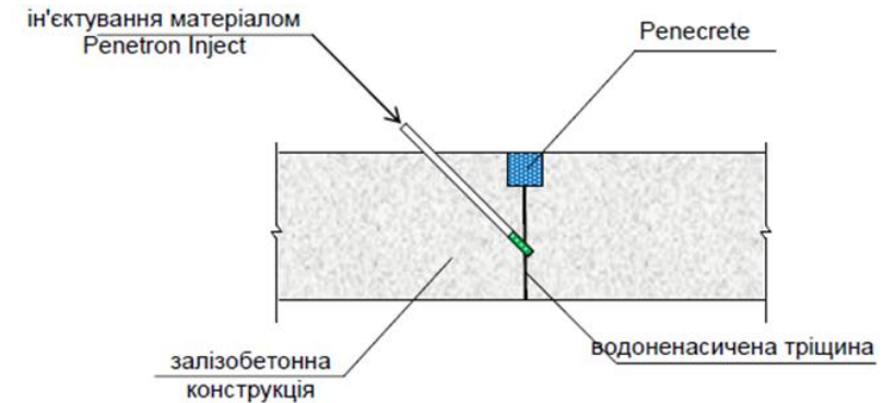
Рисунок П-9-2. Схема ін'єктування порожнин та водоненасичених статичних тріщин
