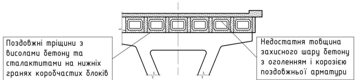
Рисунок II-7-3. Характерні пошкодження коробчастих балок
