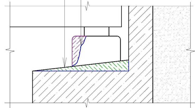
Рисунок П-8-2. Конструктивна схема ремонту підферменників
