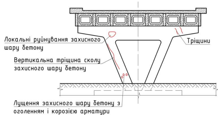
Рисунок II-6-3. Характерні пошкодження бетонної поверхні проміжних опор
