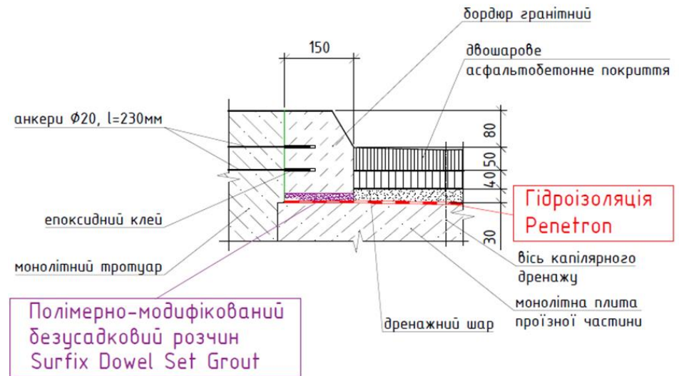
Рисунок I-2-2. Конструктивна схема улаштування гідроізоляції примикання бордюрів
