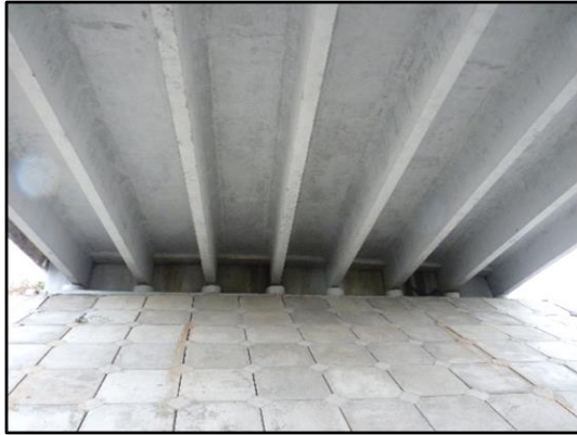
Рисунок I-4-1. Підферменники зі стічним трикутником на крайній опорі
