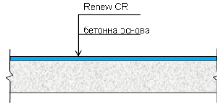
Рисунок I-12-2. Стандартна схема улаштування підлогового покриття відкритих терас, бетонних сходів та пандусів
