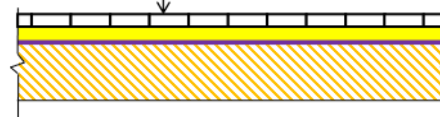
Рисунок П-14-1. Стандартна схема улаштування самонівелюючих основ (стяжок) поверх існуючих дерев'яних та плиточних підлогових основ
