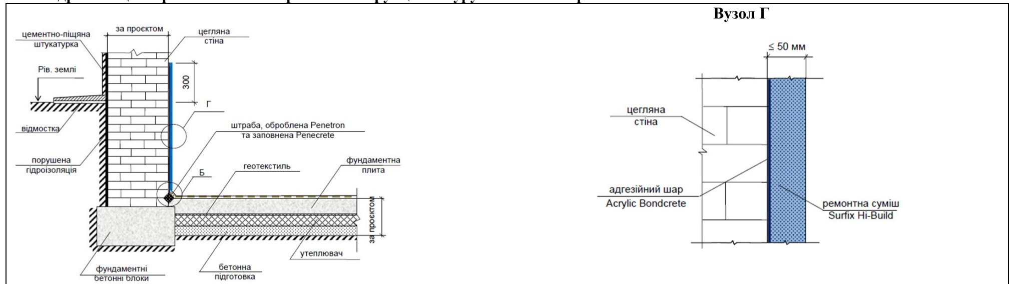
Рисунок II-3-1. Схема улаштування внутрішньої гідроізоляції вертикальних поверхонь конструкцій із муравальних матеріалів (без капілярного підсмоктування)
