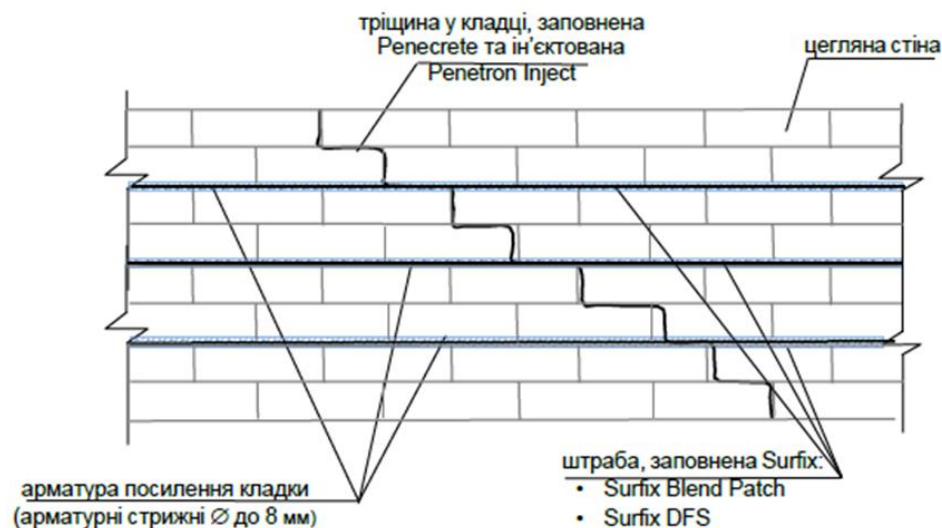
Рисунок П-7-4. Схема посилення кладки цегляної стіни
