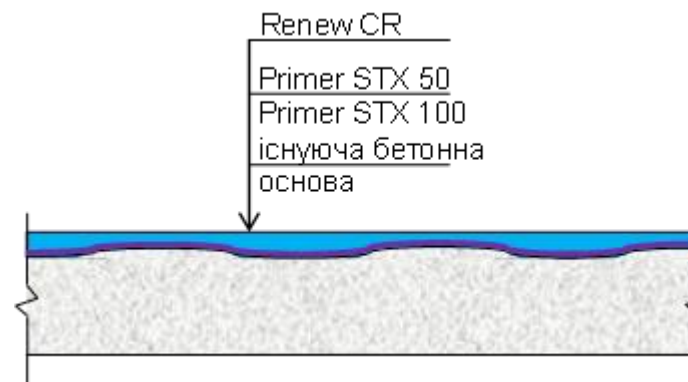
Рисунок П-11-2. Стандартна схема відновлення структурної міцності та естетичного вигляду бетонного покриття відкритих терас, бетонних сходів та пандусів
