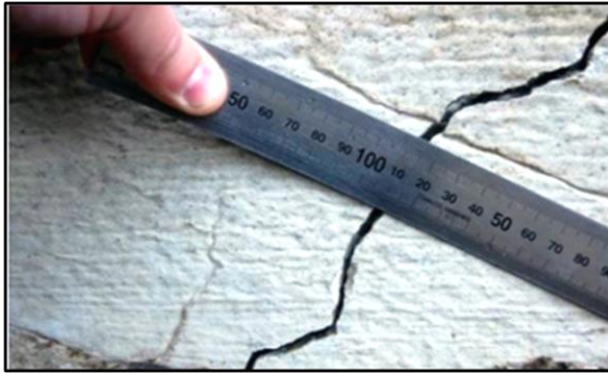
Рисунок П-8-1. Статична тріщина в залізобетонній конструкції
