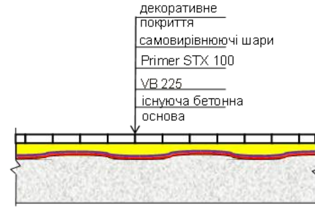
Рисунк П-13-1. Стандартна схема захисту існуючих бетонних основ, що містять підвищений рівень випаровування вологи
