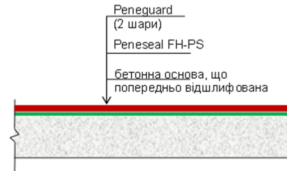
Рисунок I-13-2. Стандартна схема улаштування зносостійких полірованих підлог внутрішніх приміщень
