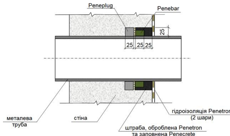
Рисунки П-4-3 і П-4-4. Схеми улаштування гідроізоляції за відсутності заповнювача або інших ущільнень між інженерними комунікаціями і металевою гільзою
