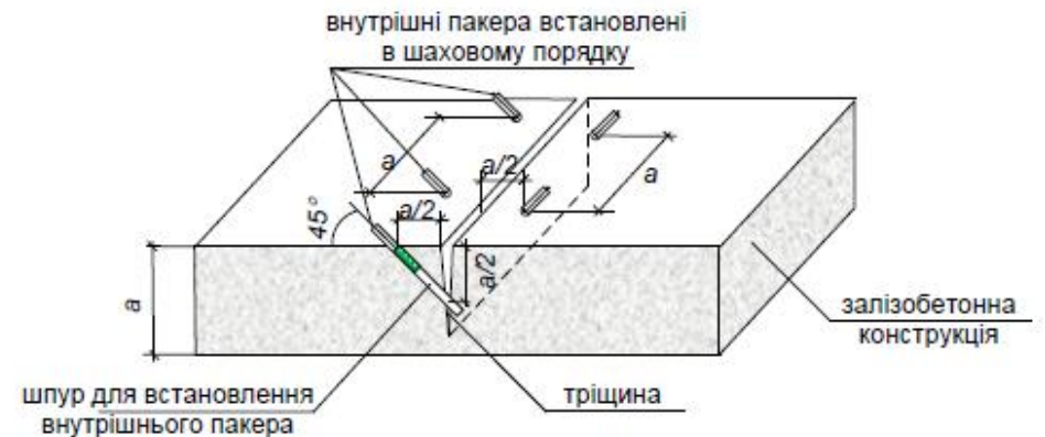
Рисунок П-8-3. Схема розташування ін'єкційних пакерів для герметизації порожнин та водоненасичених статичних тріщин
