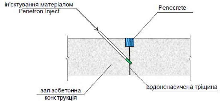
Рисунок П-8-2. Схема ін'єктування порожнин та водоненасичених статичних тріщин
