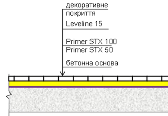
Рисунок I-14-2. Стандартна схема улаштування самонівелюючих швидкозастійшлих основ підлог внутрішніх приміщень
